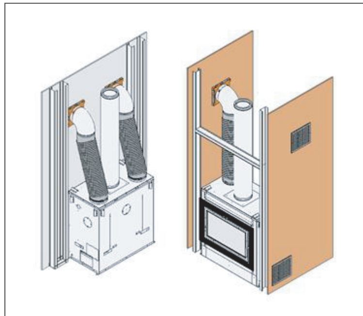
Figura 3-24: Instalación del kit de gravedad
