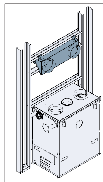
Figura 3-26: Instalación del adaptador de conducto/rejilla lineal
