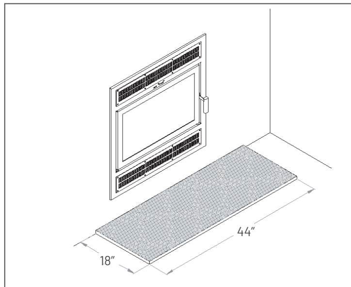
Figura 3-37: Extensión del hogar
