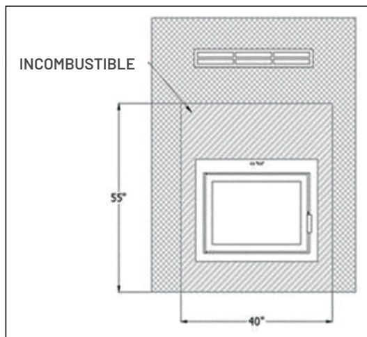
Figura 3-41: Compartimiento frontal para la configuración de marco liso con rejilla lineal
