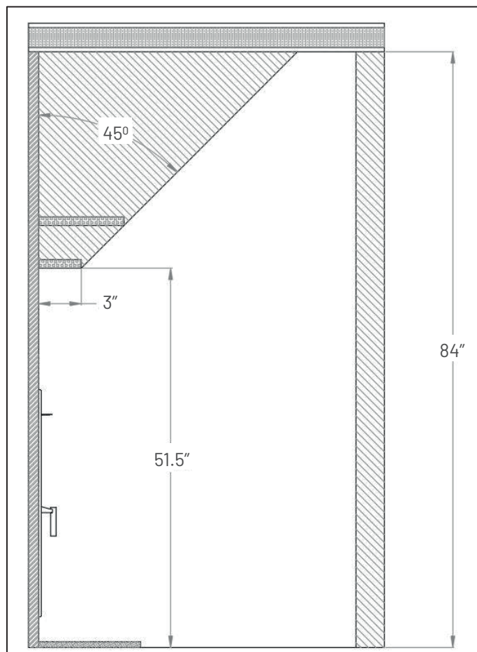
Figura 3-42: Espacio libre de la repisa
