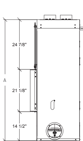
Vista lateral
