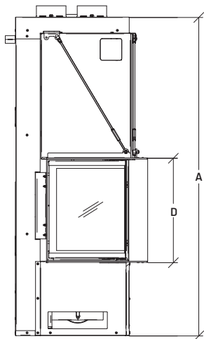
Vista lateral
